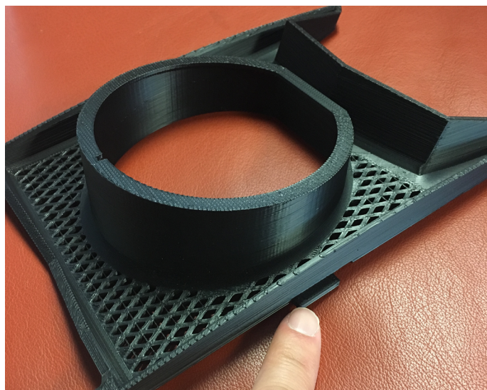
Figure 5. Languettes du support de relocalisation
