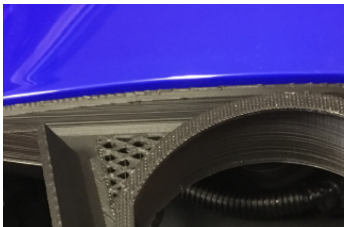
Figure 12. Positionnement incorrect du support de relocalisation
