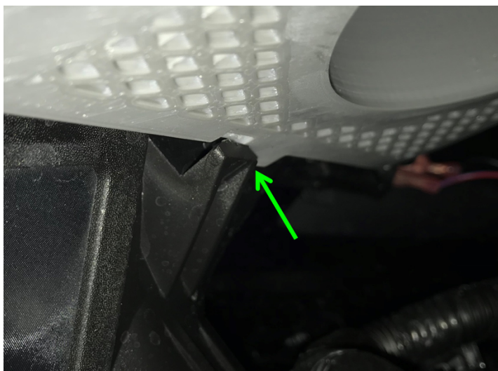
Figure 13. Positionnement correct du support de relocalisation, vue du dessous
