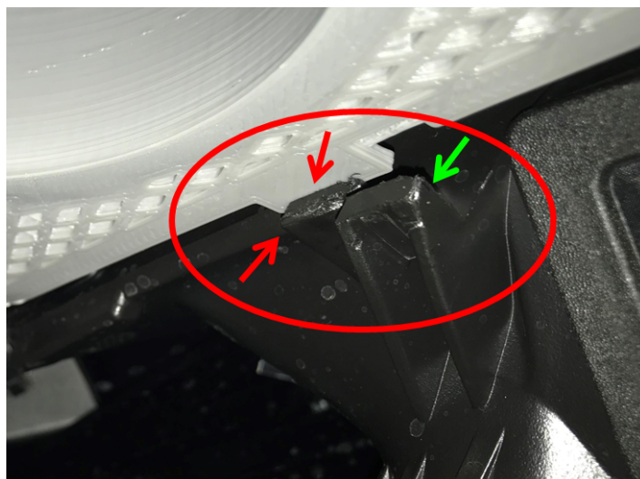
Figure 14. Positionnement incorrect (appui languette supérieure) du support de relocalisation, vue du dessous
