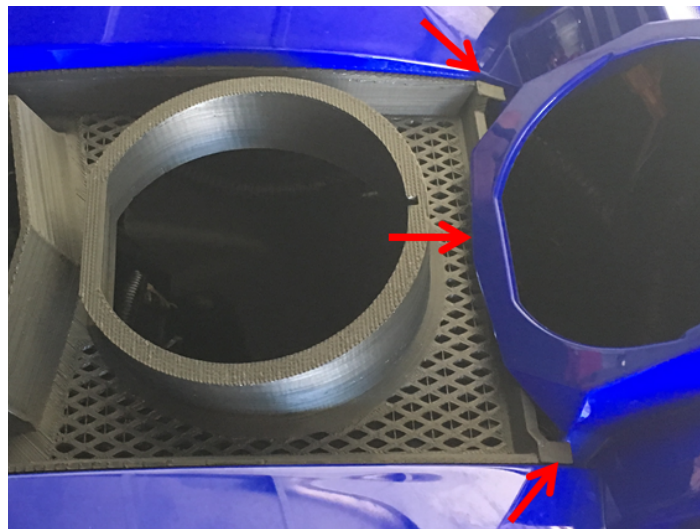
Figure 10. Positionnement final du support de relocalisation 2
