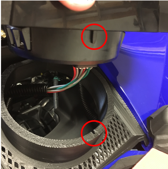
Figure 16. Combiné d'instruments installé
